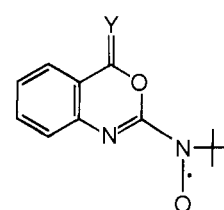
63a 135 Y = O, NC(CH 3 ) 3
